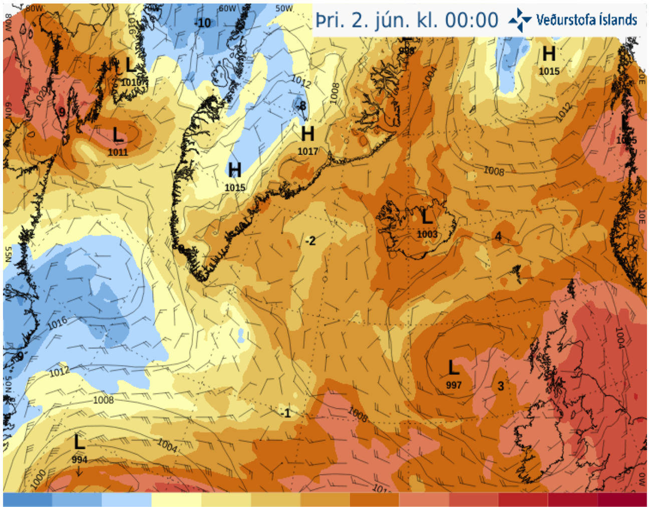
Hiti í 850 hPa (°C), vindur í 100 m hæð og loftþrýstingur (hPa) ECMWF/ECM 0.125: 01.06.2026 00:00 UTC (+24)
